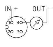
1 (IN) 4 (OUT)
